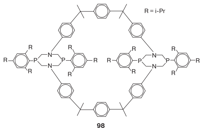
Рис. 36. Схема и ключевые скалярные корреляции для макроцикла 98.
