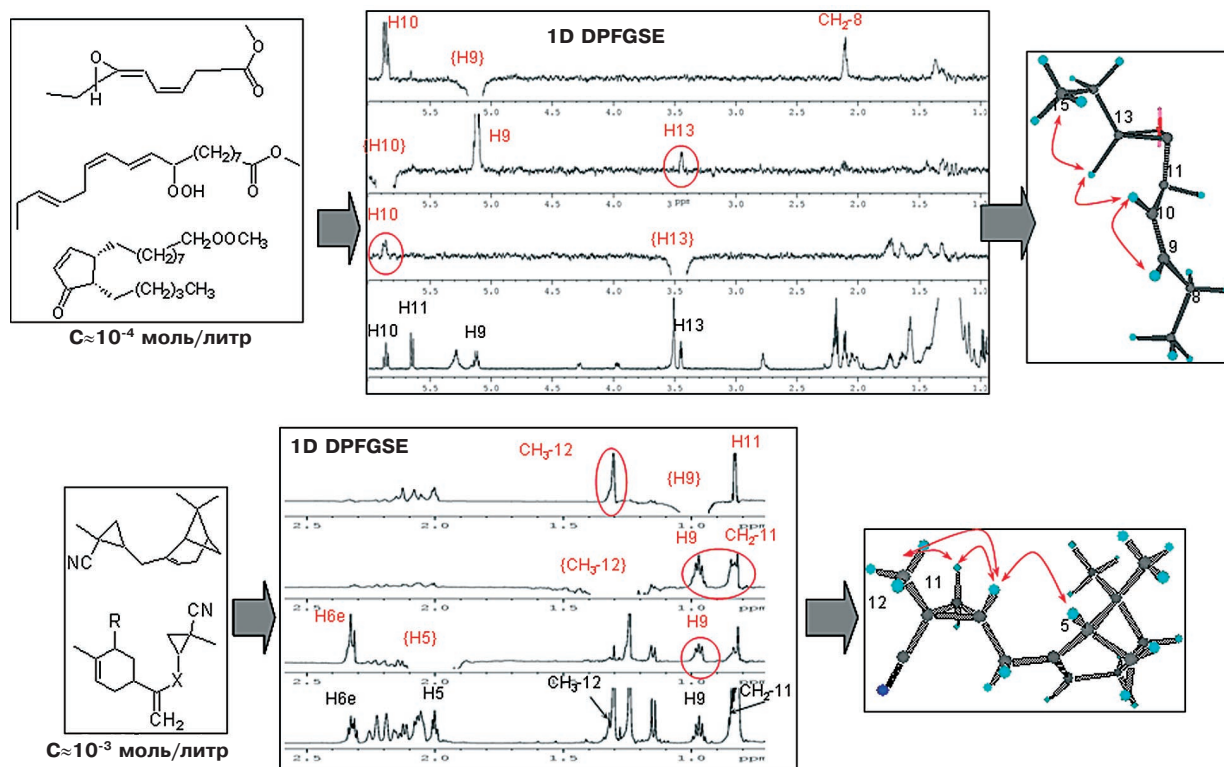
Рис. 23. 1D DPGSE спектры 57 и 60 , принципиальные ЯЭО и их корреляции со структурой.
