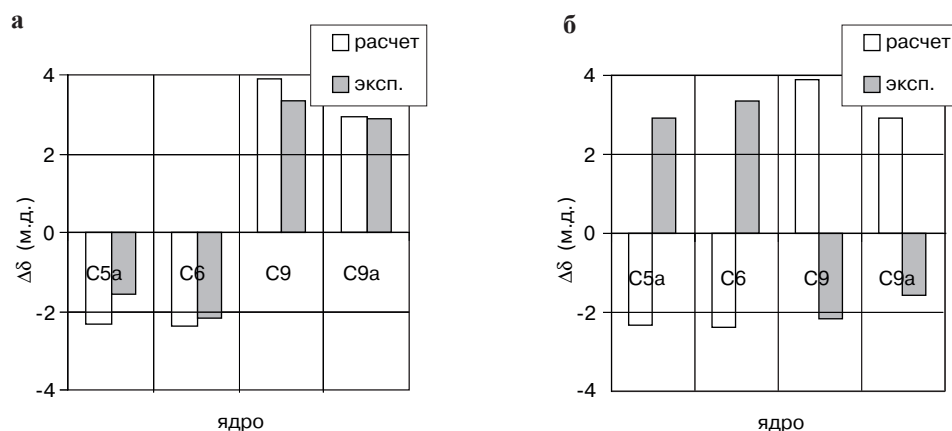
Рис. 15. Разница экспериментальных и расчетных ХС ^{13}\text{C} ( \Delta\delta , м.д.) для различных отнесений изомерной структуры 19 и 20 : а \Delta\delta = \delta_{i_{\text{exp.1}}} - \delta_{i_{\text{exp.2}}} vs. \Delta\delta = \delta_{i_{\text{calc.1}}} - \delta_{i_{\text{calc.2}}} , б \Delta\delta = \delta_{i_{\text{exp.1}'}} - \delta_{i_{\text{exp.2}'}} vs. \Delta\delta = \delta_{i_{\text{calc.1}}} - \delta_{i_{\text{calc.2}}} .
