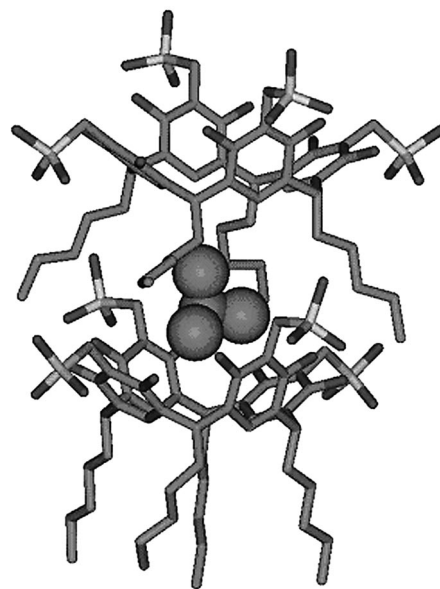
Рис. 33. Структура субъединицы в агрегатах сульфатный каликс[4]резорцинарен + тетраметиламоний.
