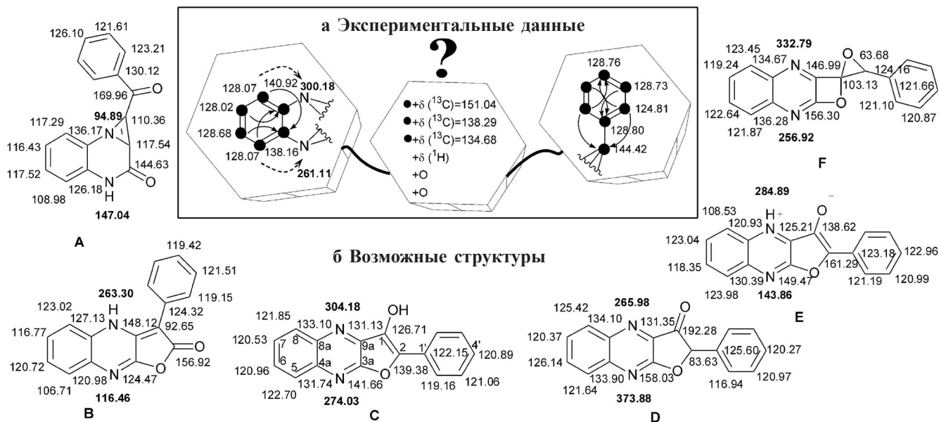
Рис. 14. а Экспериментальные данные: принципиальные HMBC корреляции (от протонов к углеродам – сплошные стрелки и к азотам – штрихованные стрелки) и ХС ^{13}\text{C} и ^{15}\text{N} соединения; б возможные структурные изомеры соединения 16 с рассчитанными ХС ^{13}\text{C} и ^{15}\text{N} (жирный шрифт).
