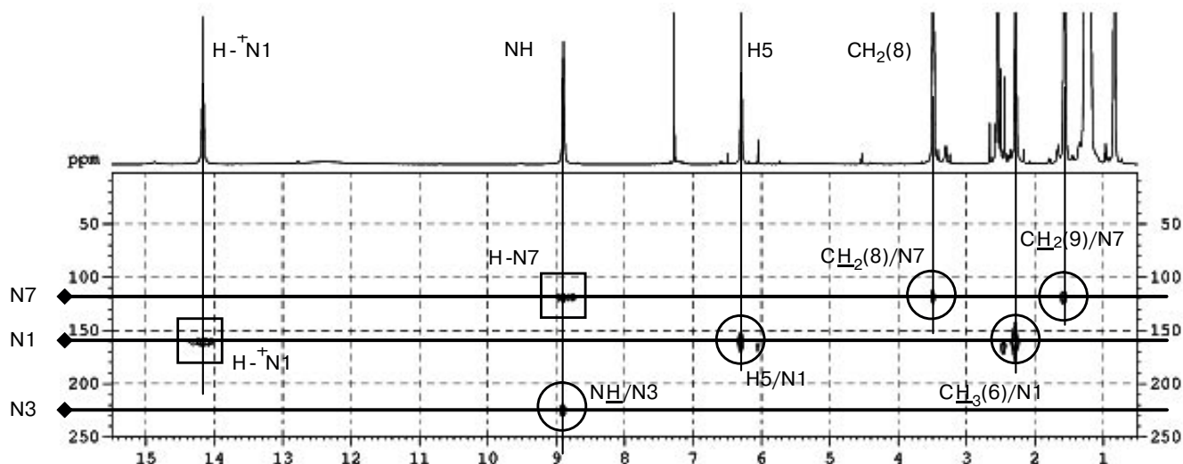
Рис. 19. Суперпозиция ^1\text{H} - ^{15}\text{N} HSQC (кросс-пики в квадратах) и ^1\text{H} - ^{15}\text{N} HMBC (кросс-пики в кружках) спектров протонированной формы соединения 56 при T = 233 K.
